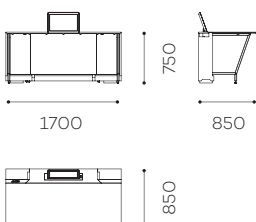
Open module
