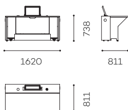
Open module
