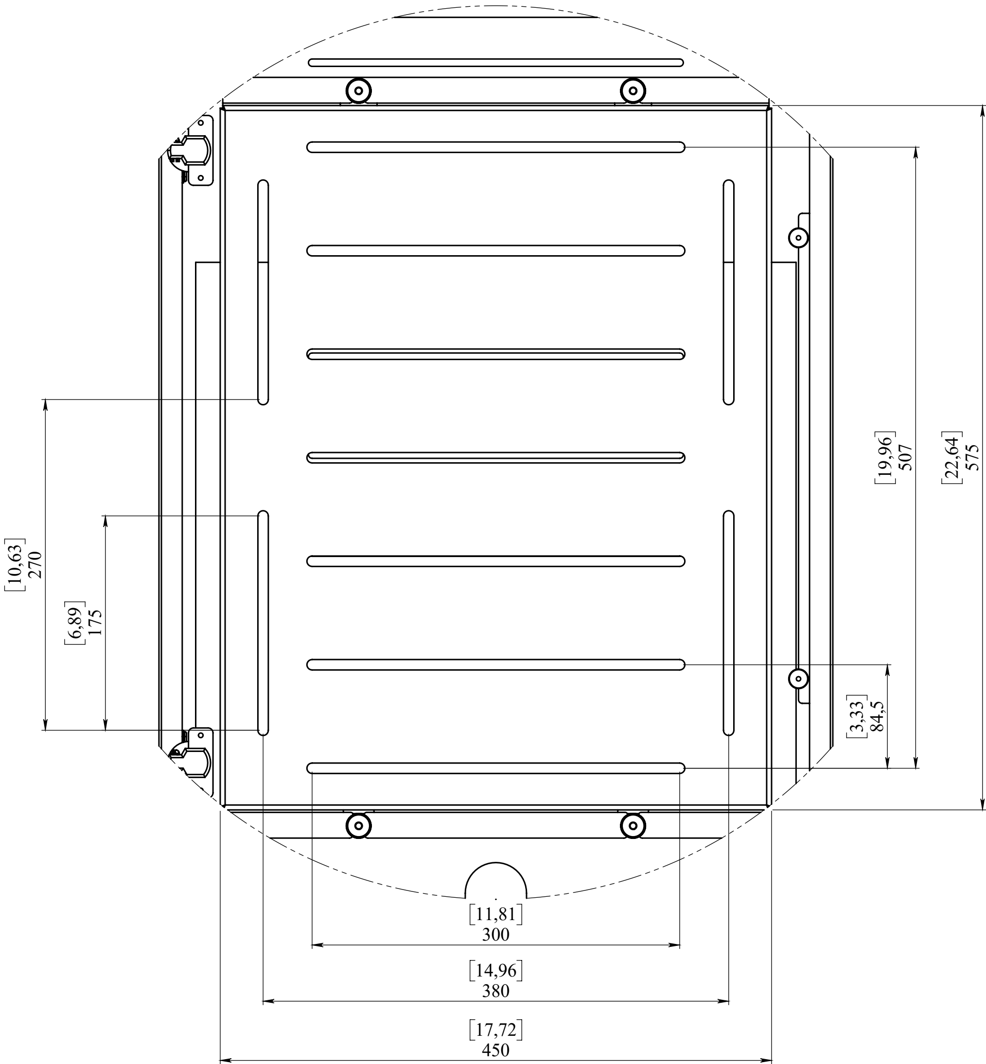
DÉTAIL B ECHELLE 1 : 3
