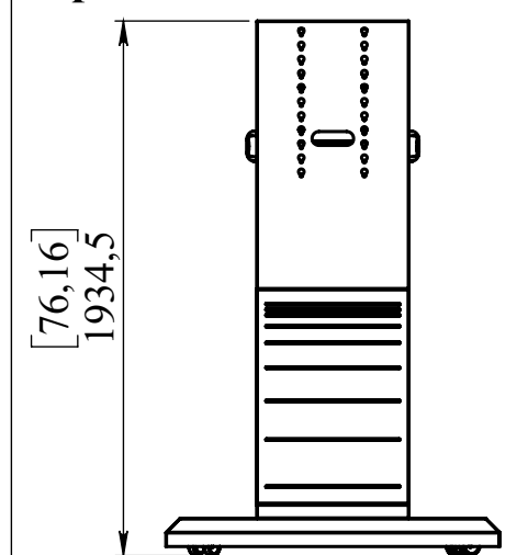
Option : Roulettes Ø100
