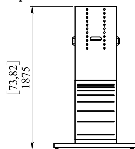
Option : Roulettes Ø35
