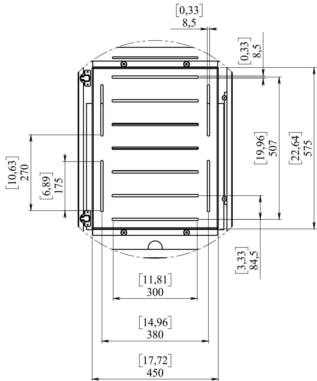
DÉTAIL B ECHELLE 1 : 8
